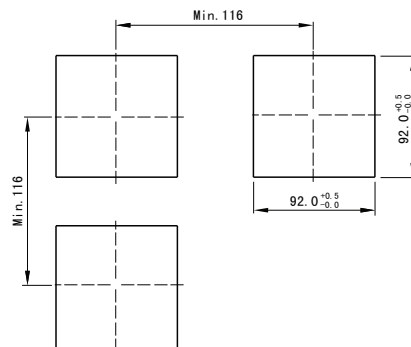
开孔尺寸
