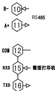
通讯及微型打印机接线图
