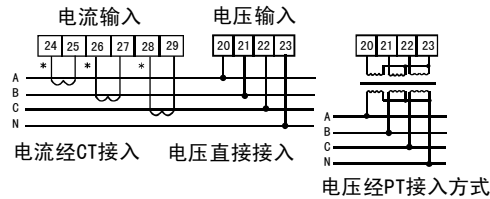
方式1 (3个CT) : 三相四线的接线方式
